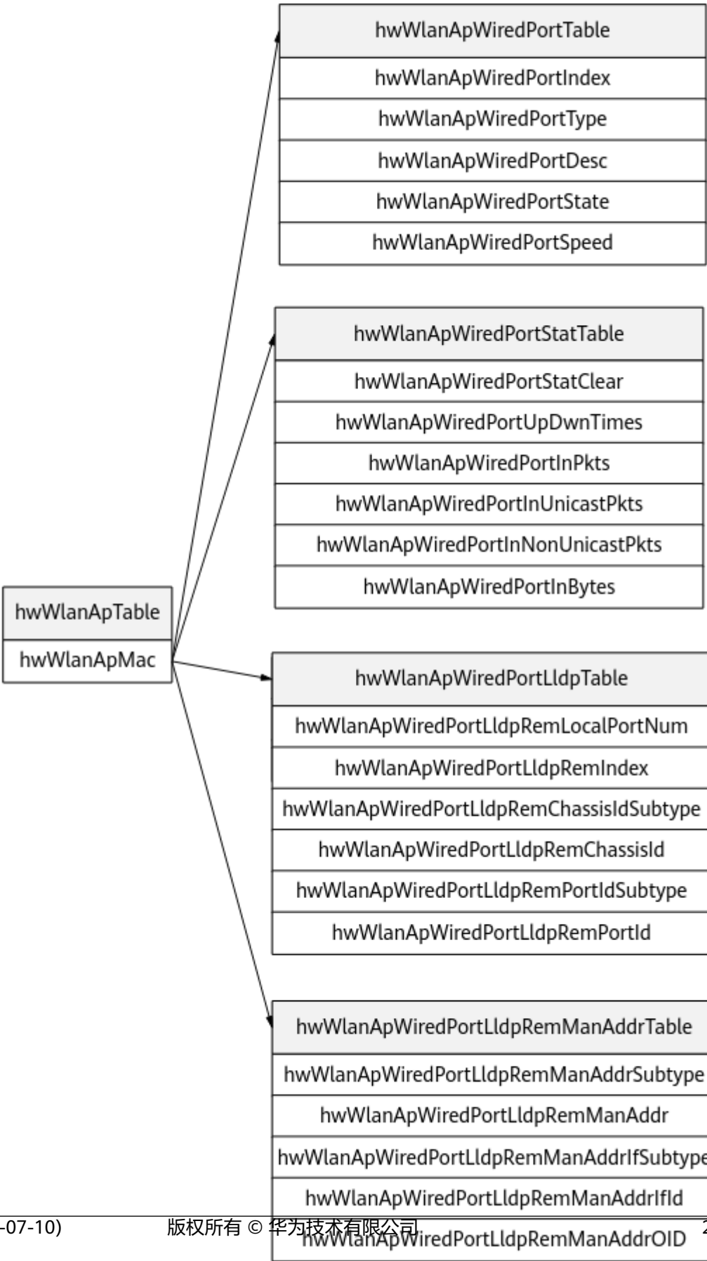
图 143-1 hwWlanApTable、hwWlanApWiredPortTable、hwWlanApWiredPortStatTable、hwWlanApWiredPortLldpTable 和 hwWlanApWiredPortLldpRemManAddrTable 的表间关系
