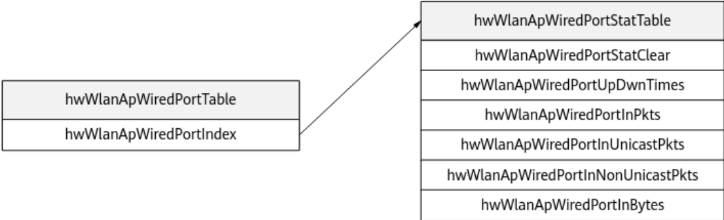
图 143-2 hwWlanApWiredPortTable 和 hwWlanApWiredPortStatTable 的表间关系
