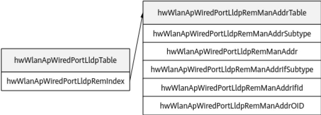
图 143-3 hwWlanApWiredPortLldpTable 和 hwWlanApWiredPortLldpRemManAddrTable 的表间关系
